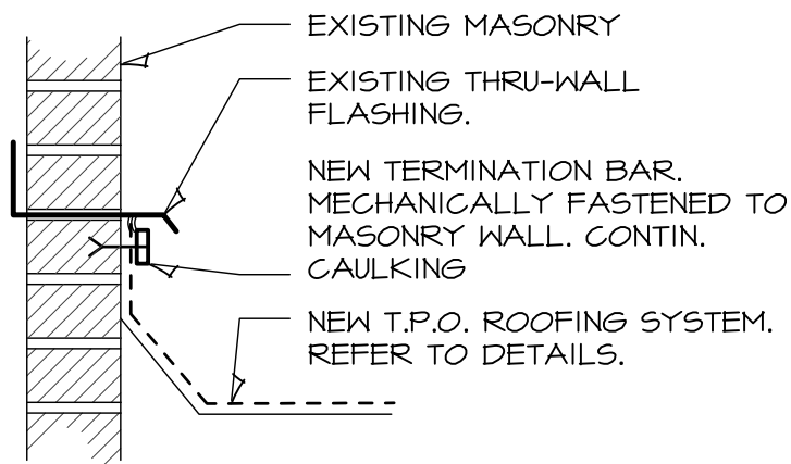
DETAIL - N.T.S.
